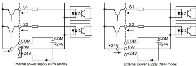
Рис. 4-22 Режим NPN
