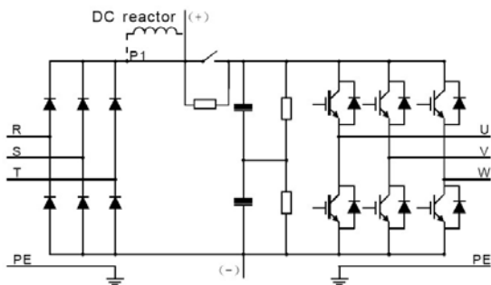
Рис. 3-1 Схема силовой цепи (≤30кВт)
