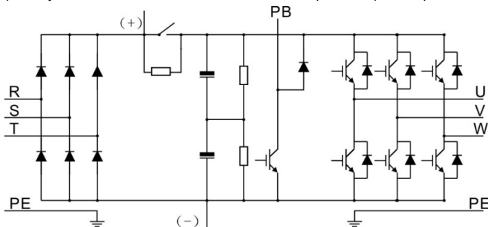
Рис. 3-1 Схема силовой цепи (≤30кВт)
