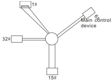
Рис. 10. 5 Подключение «Звезда»
